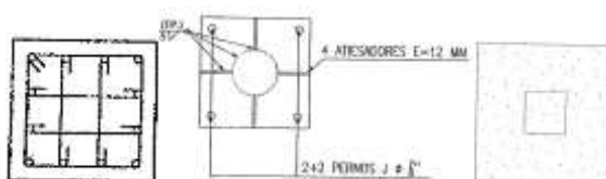
Detalle pedestal, placa base y planta fundación referencial.
