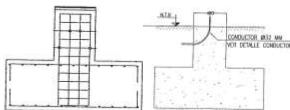
Detalle armadura y elevación fundación referencial.
